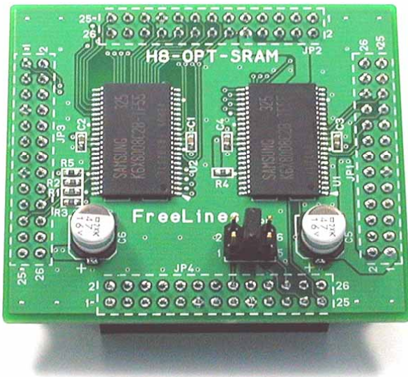
【弊社製 H8 評価ボードと組み合わせた写真】
